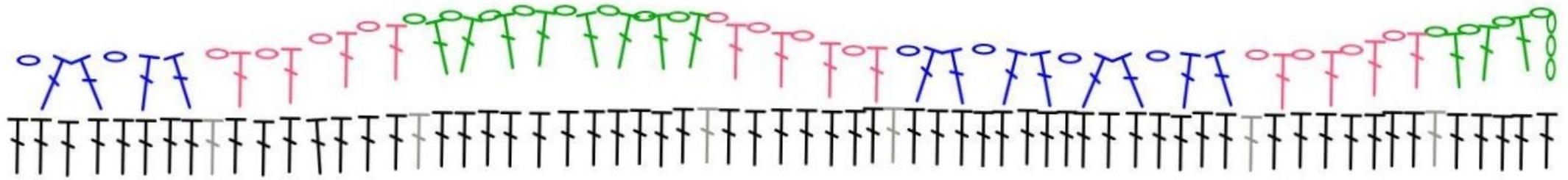
Waves - Vlny - 1
